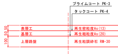
施工要領図
